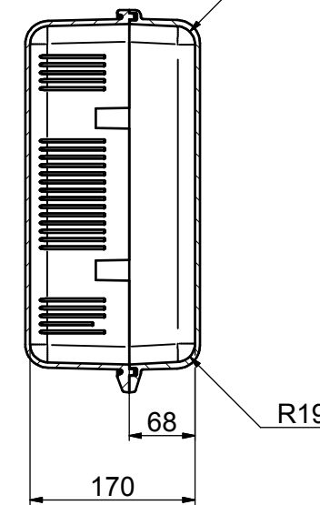
A-A (1:5)
